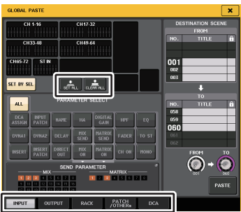
Окно GLOBAL PASTE (Глобальная вставка)
