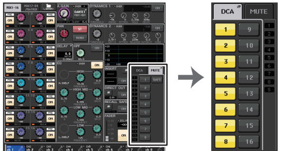
SELECTED CHANNEL (Выбранный канал) Экран VIEW Поле DCA/MUTE (DCA/приглушение)
